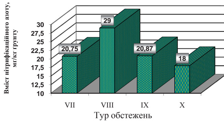
Рис. 6. Динаміка вмісту азоту (за нітрифікаційною здатністю ґрунту, мг/кг) в зрошуваній сівозміні №1 ДГДГ "Асканійське" за турами обстежень (1997-2010 рр.)
