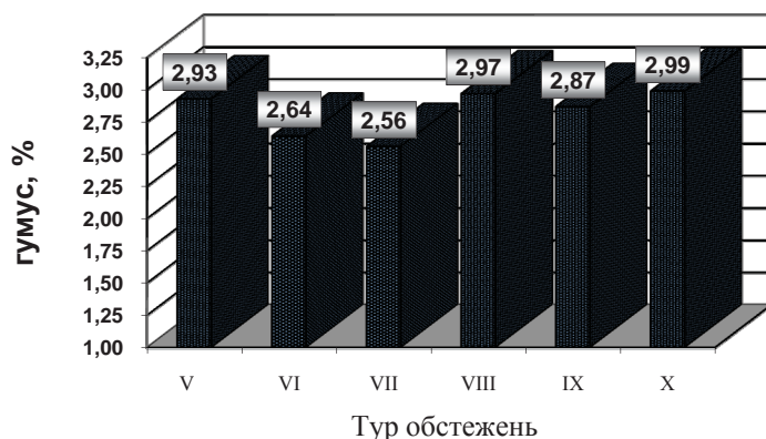
Рис. 4. Динаміка вмісту гумусу на чорноземах південних польової зрошуваної сівозміни № 1 ДПДГ "Асканійське" за турами обстежень (1986-2010 рр.)
