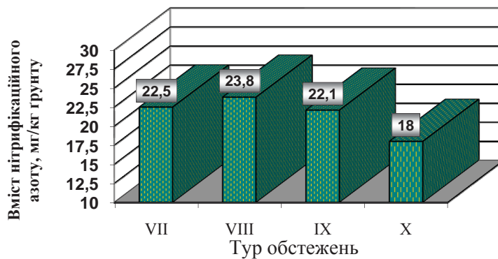
Рис. 7. Динаміка вмісту азоту (за нітрифікаційною здатністю ґрунту, мг/кг) в зрошуваній сівозміні №3 ДГДГ "Асканійське" за турами обстежень (1997-2010 рр.)
