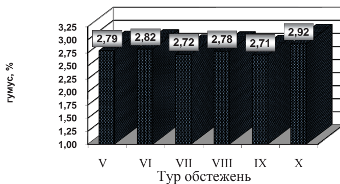
Рис.5. Динаміка вмісту гумусу на темно-каштанових ґрунтах польової зрошуваної сівозміни № 3 ДПДГ "Асканійське" за турами обстежень (1986-2010 рр.)
